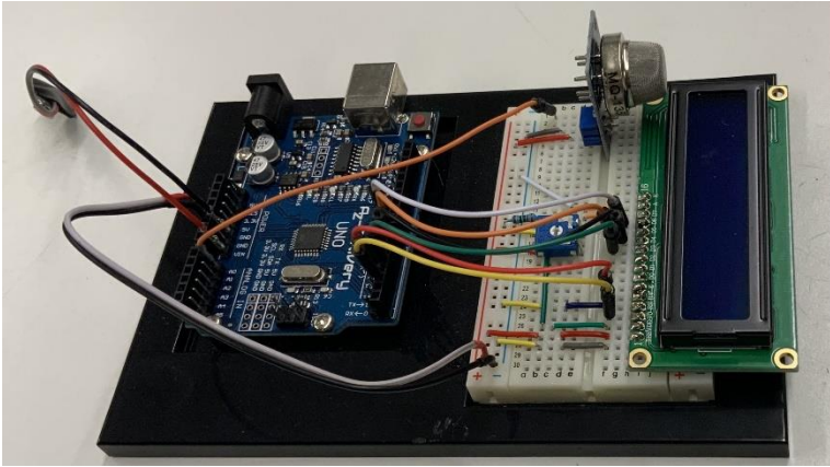
Prototyp mit LCD des Luftqualitätsmessgeräts im Selbstbau des Gymnasiums Süderelbe
